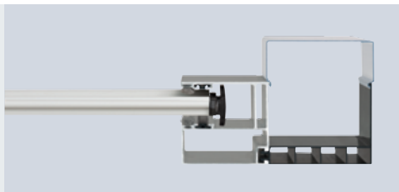
Perfil Decotherm S de una puerta enrollable SB / TGT con gancho antitormenta de material sintético
