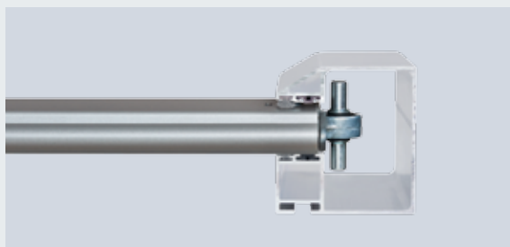
Perfil HR 116 A de una puerta enrollable DD con gancho antitormenta de acero
